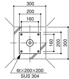
A - A' 平面図
