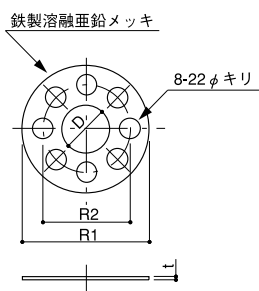
支線、架空地線用引留ディスクプレート
