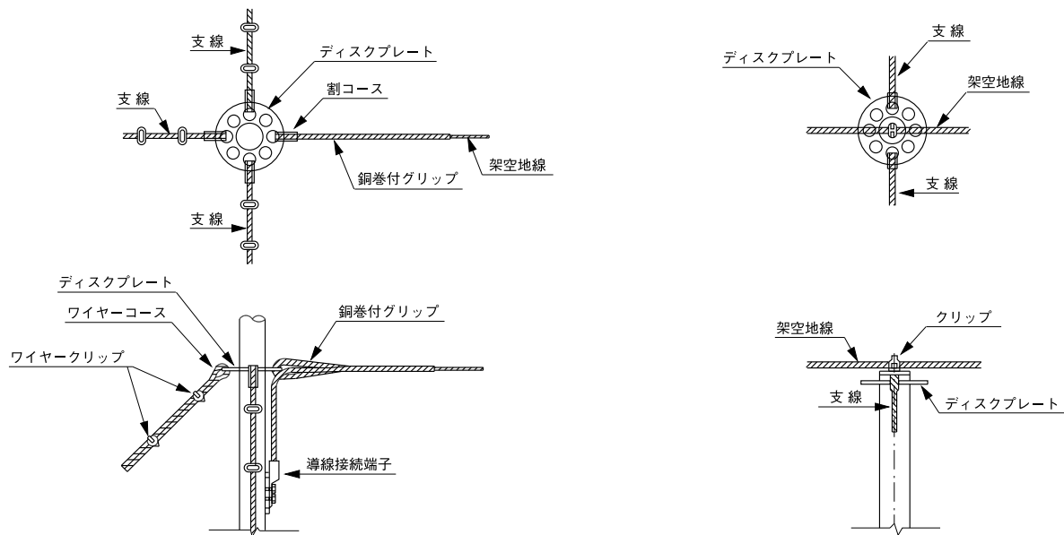
A部詳細
