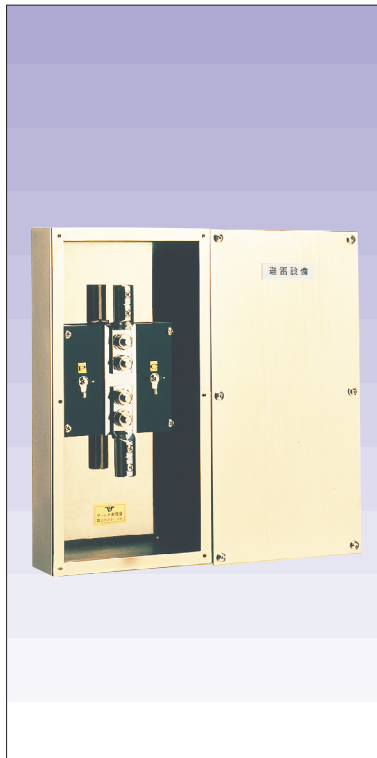
試験用端子函国土交通省仕様TB-ASIA露出型 (黄銅製ホワイトブロンズメッキ仕上) 品番 641
